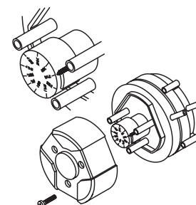
Suodatinvahti, paine-erokytkin
